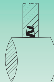
Obturación de NBR "ZF" para: SN "ZF" NBR seal for: SN
