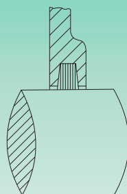
Obturación de fieltro "TSNC" para: SNG-SNU "TSNC" felt seal for: SNG-SNU
